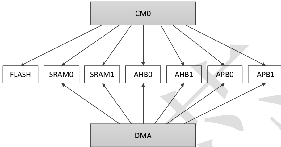
图 3 LCM32A039C8T8 总线矩阵
