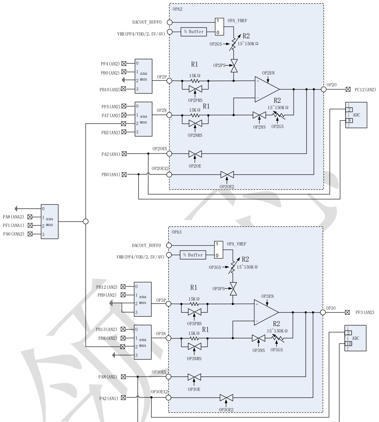
图 7 OPA 内部结构和外部互联
