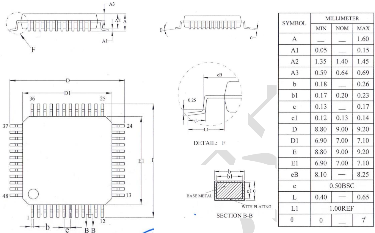
图 11 LQFP48 (7*7-P0.5) 封装尺寸
