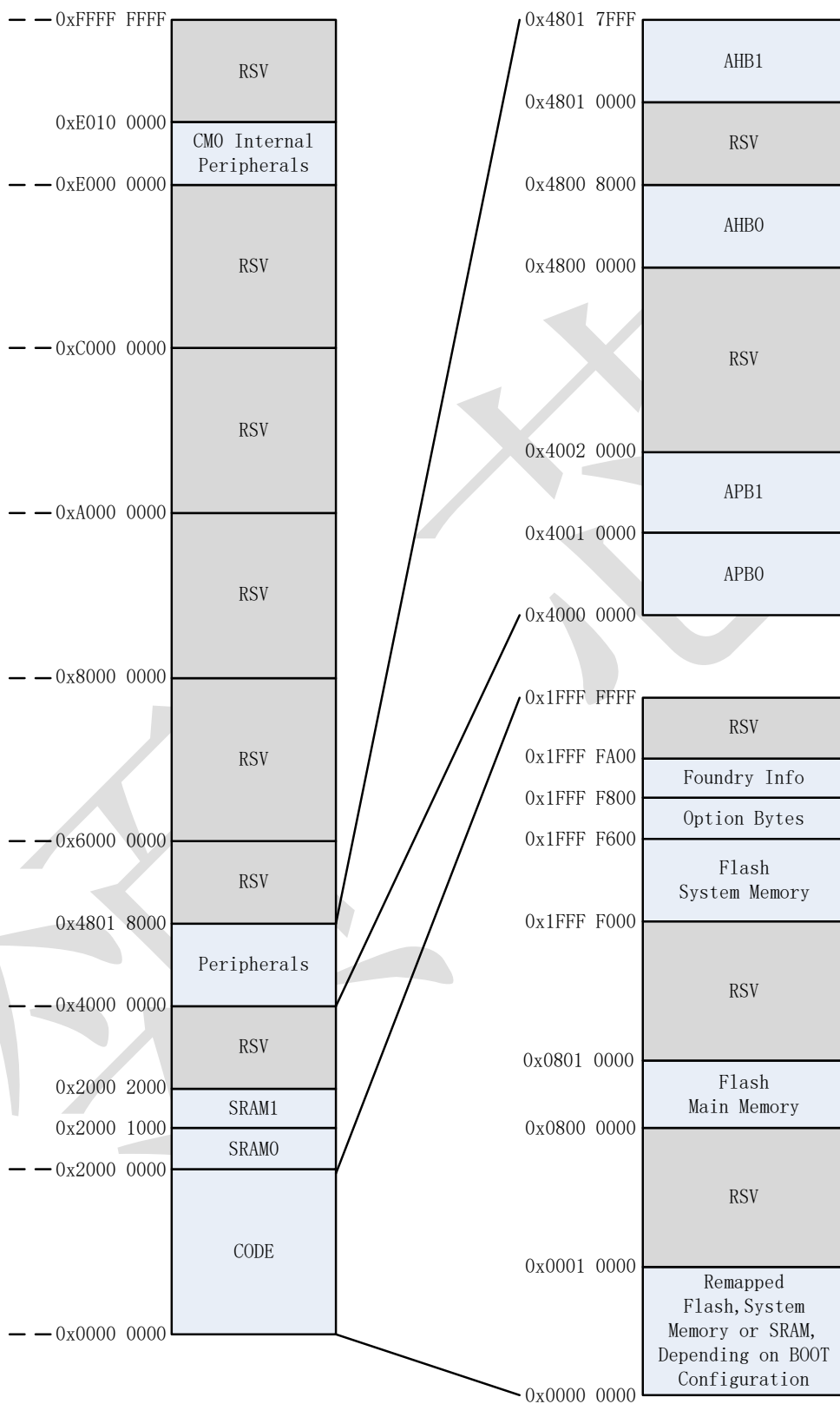
图 10 LCM32A039C8T8 存储器映射
