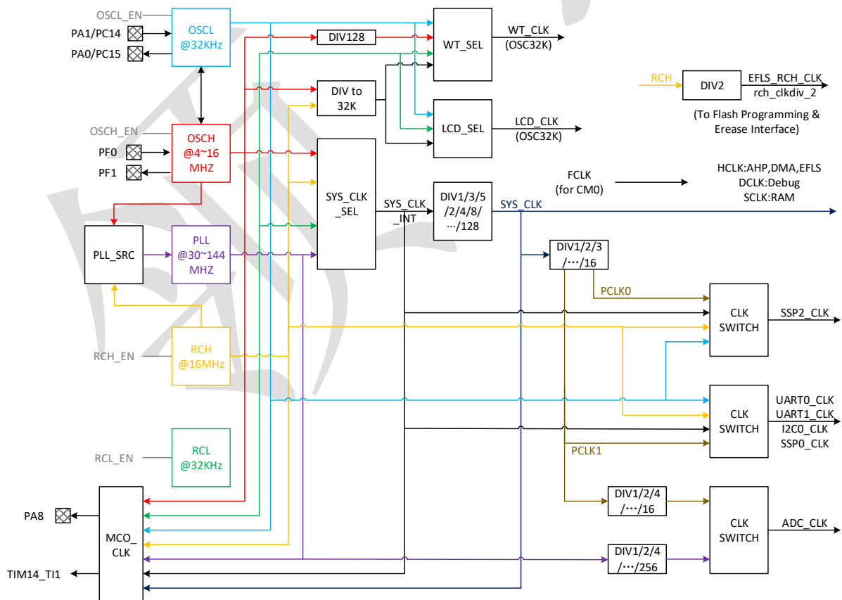
图 2 LCM32A039C8T8 时钟树
